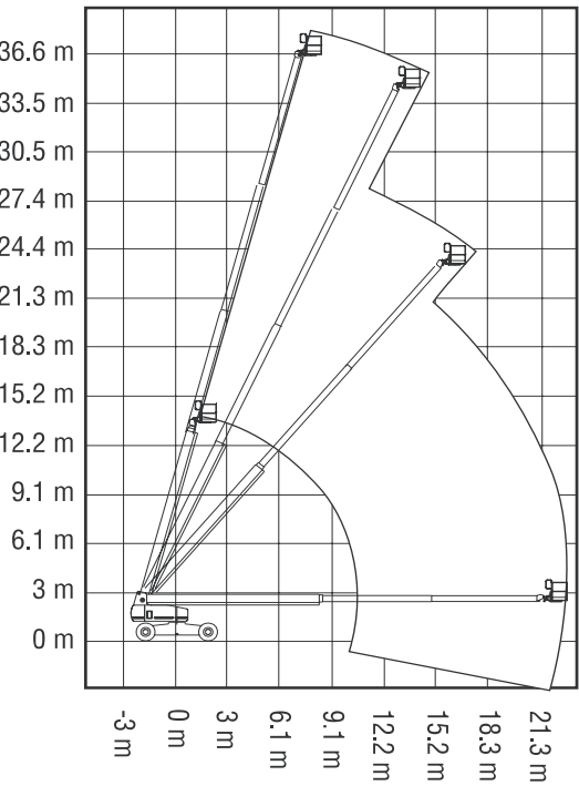
S-120 运动范围表
