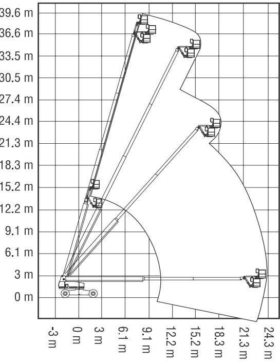
S-125 运动范围表
